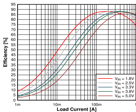
图 9-4. Efficiency
