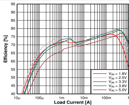
图 9-3. Efficiency
