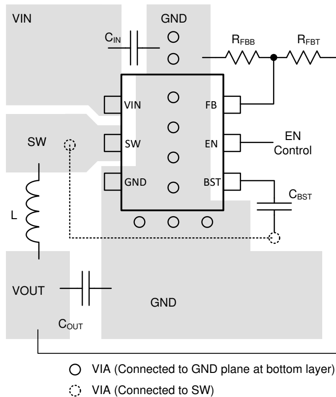
图 11-1. TPS562207S Layout
