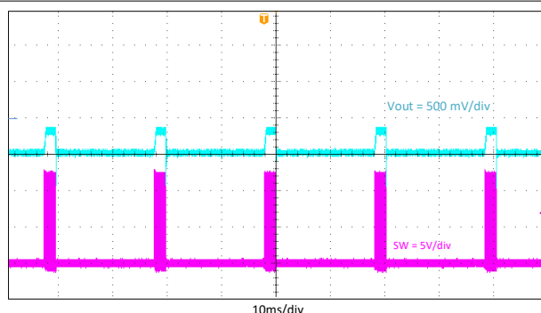
图 9-7. Hiccup, I_{out} = 5\text{ A}
