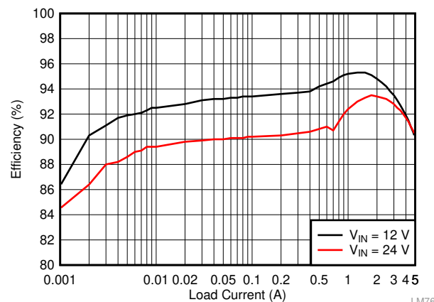
效率: V_{OUT} = 5V , f_{sw} = 400kHz , 自动模式
