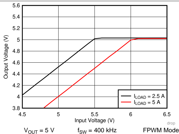
图 20. LM76005 Voltage Dropout
