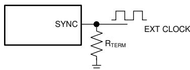
图 12. Frequency Synchronization
