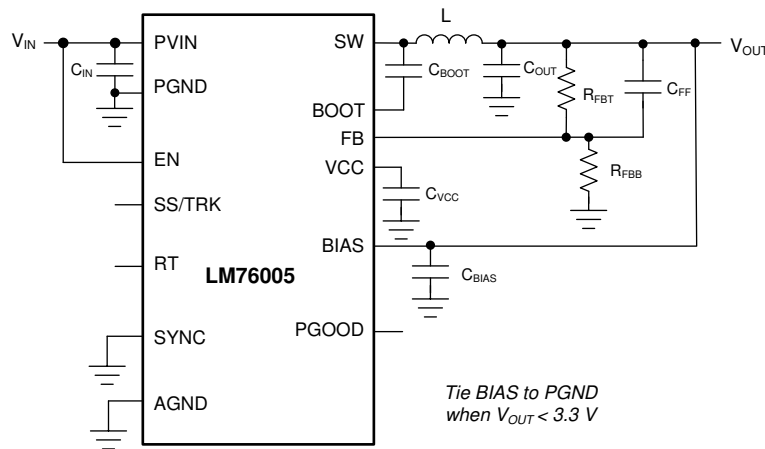
图 15. LM76005 Basic Schematic
