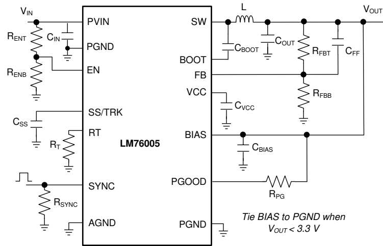
图 16. LM76005 Comprehensive Schematic
