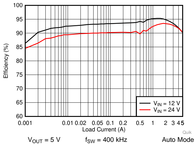
图 18. LM76005 Efficiency
