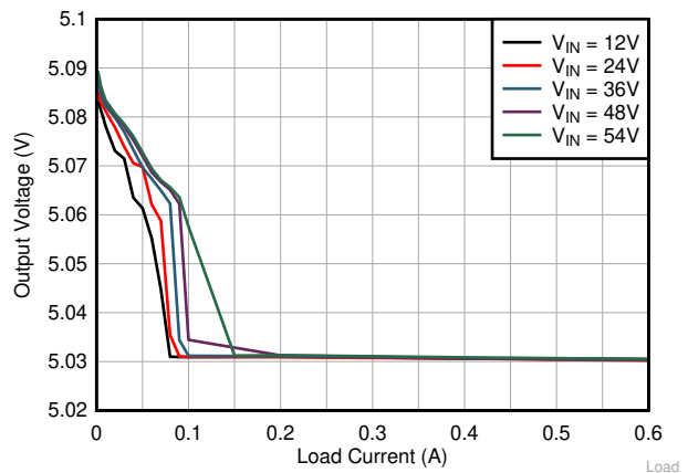
LMR36506R V_{OUT} = 5 V 400 kHz (AUTO)
