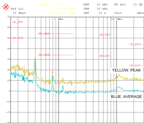
LMS3655-Q1 传导 EMI: 输出电压 = 5V, 输出电流 = 5A
