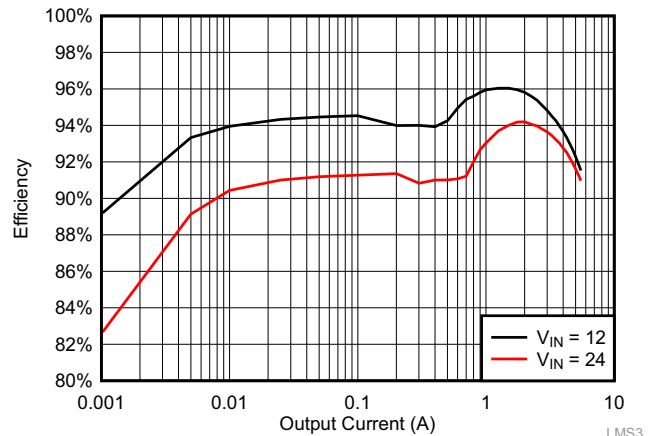
LMS3655-Q1 效率: 输出电压 = 5V
