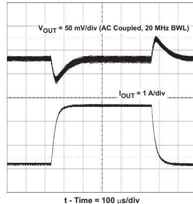
图 15. Transient Response
