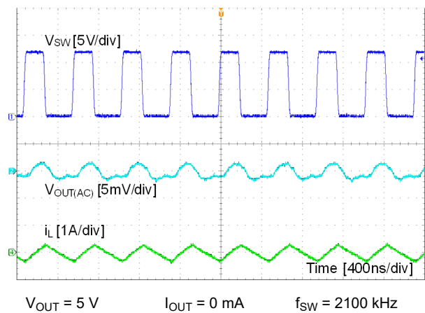
图 8-5. FPWM Mode
