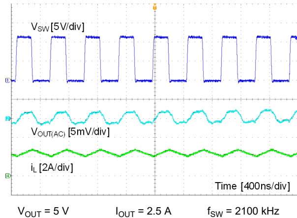
图 8-2. CCM Mode
