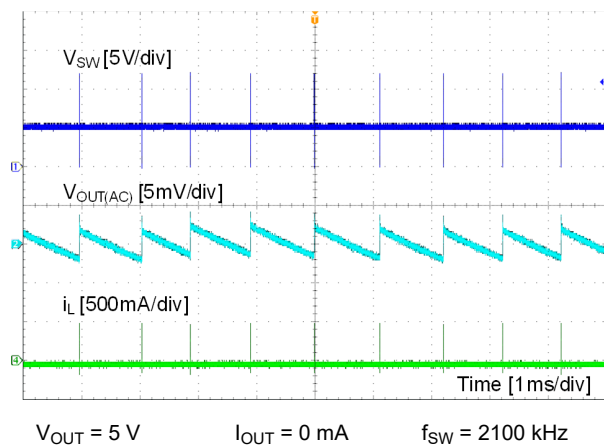
图 8-4. PFM Mode
