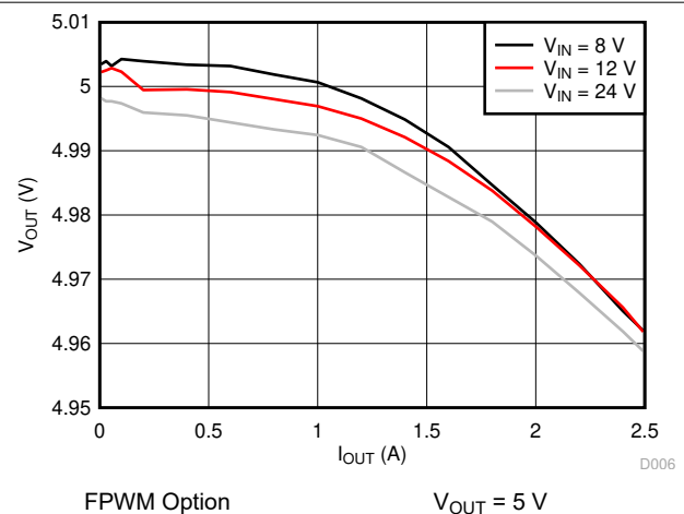
图 6-6. Load Regulation
