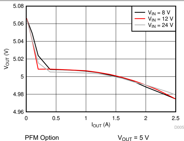
图 6-5. Load Regulation
