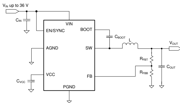
简化原理图
