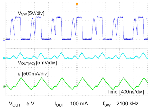
图 8-3. DCM Mode
