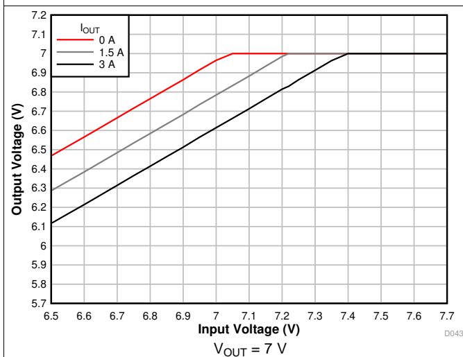
图 35. Voltage Dropout
