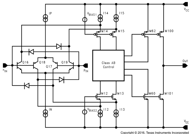
简化原理图
