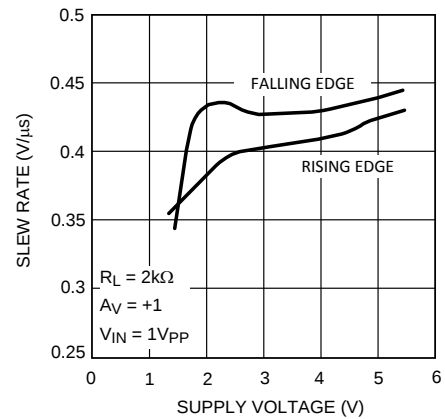
Figure 16. 压摆率与电源电压间的关系
