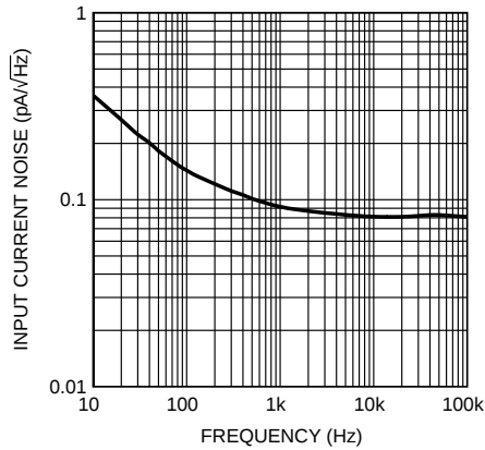
Figure 13. 输入电流噪声与频率间的关系
