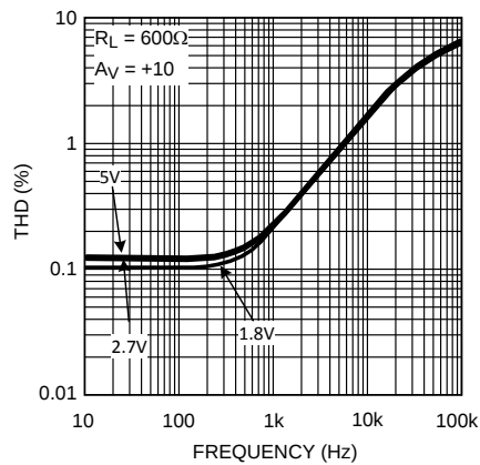
Figure 15. THD 与频率间的关系
