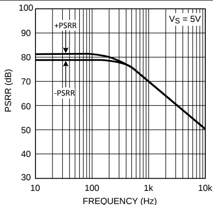
Figure 11. PSRR 与频率间的关系
