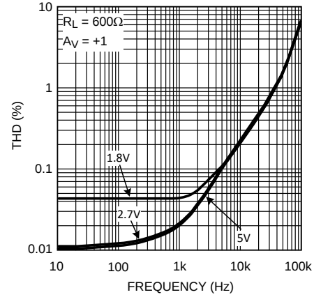
Figure 14. THD 与频率间的关系
