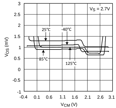
Figure 26. 失调电压与共模范围间的关系
