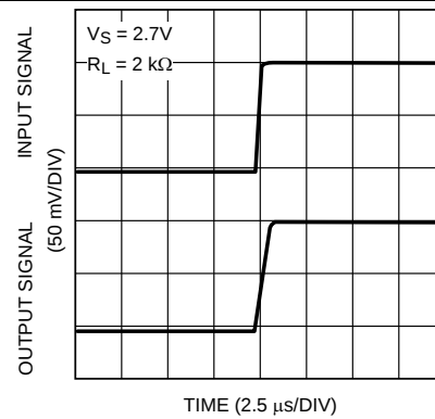
Figure 18. 小信号同相响应
