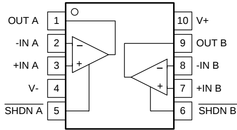
引脚功能：LMV982-N
