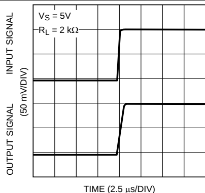
Figure 19. 小信号同相应
