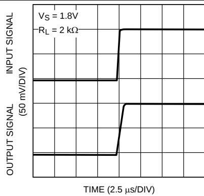
Figure 17. 小信号同相响应
