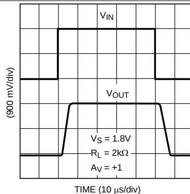
Figure 20. 大信号同相应
