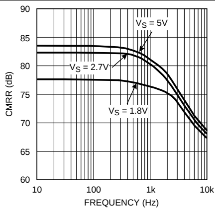
Figure 10. CMRR 与频率间的关系
