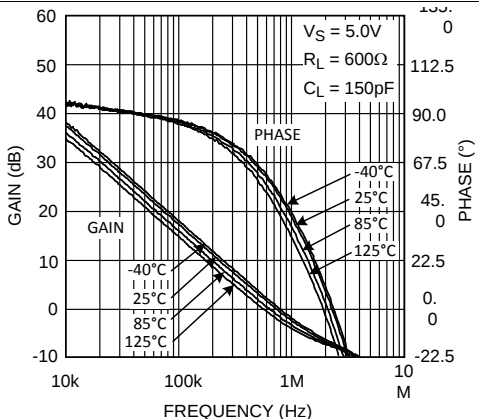
Figure 9. 增益和相位与频率间的关系
