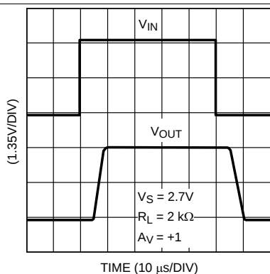
Figure 21. 大信号同相应
