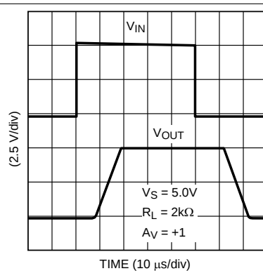
Figure 22. 大信号同相应
