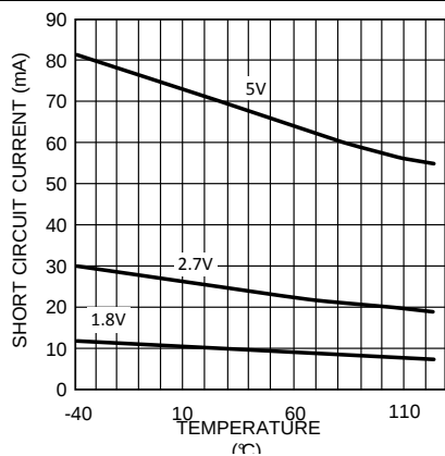
Figure 23. 短路电流与温度间的关系（灌电流）
