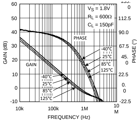
Figure 8. 增益和相位与频率间的关系
