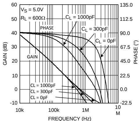
Figure 7. 增益和相位与频率间的关系
