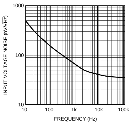
Figure 12. 输入电压噪声与频率间的关系
