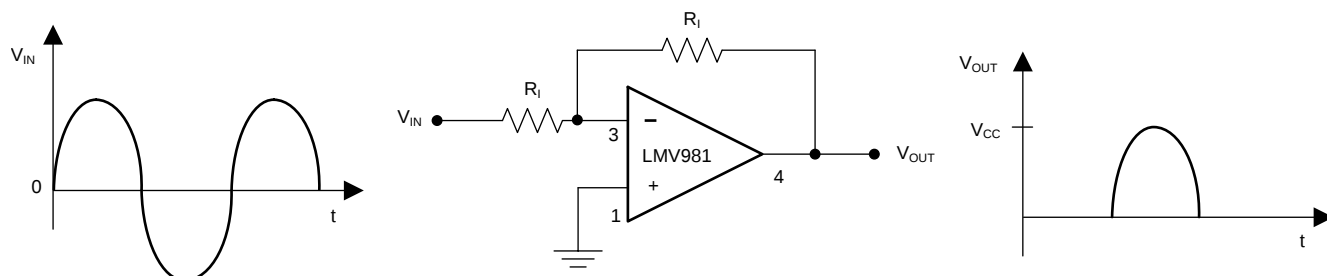
Figure 32. 半波整流器的轨至地输出摆幅以地为参考
