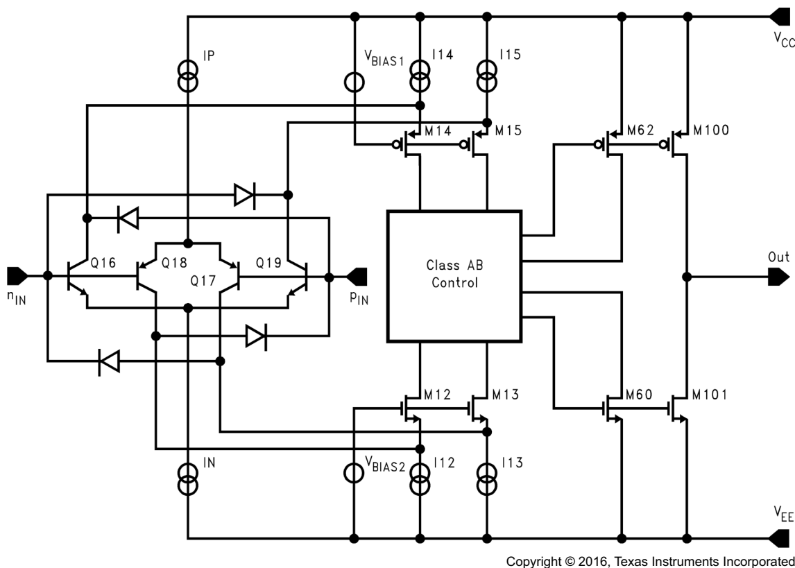
Figure 28. 简化原理图
