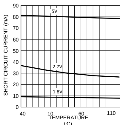
Figure 24. 短路电流与温度间的关系（拉电流）
