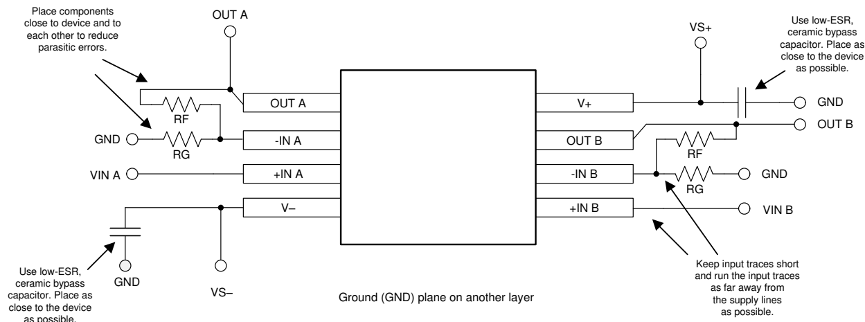
图 37. Layout Example
