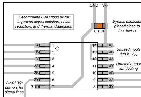
图 11. Example layout for the SN74HCS32-Q1
