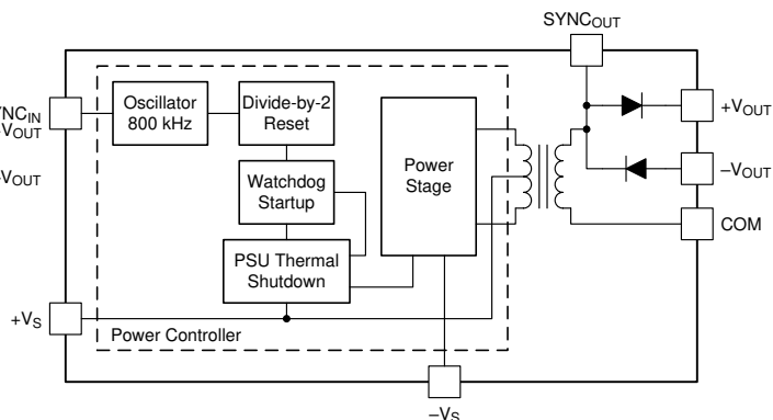
双路输出方框图
