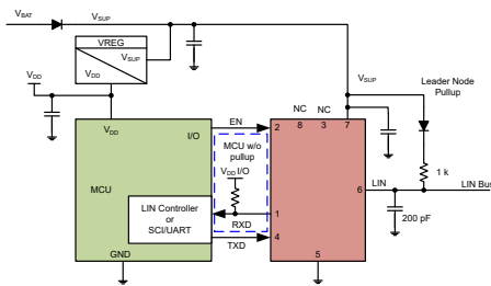
简化原理图，领导模式 (1)
