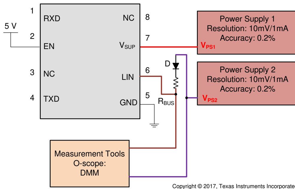
图 8-5. V<sub>SUP</sub>_NON_OP Param 11
