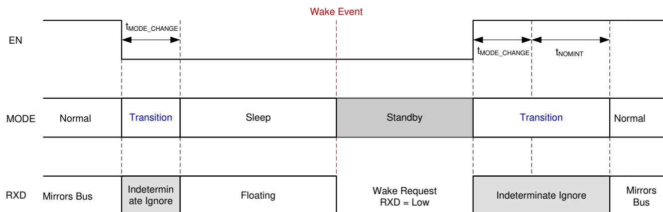
图 8-15. Mode Transitions
