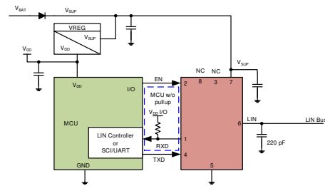
简化原理图，跟随者模式 (2)
