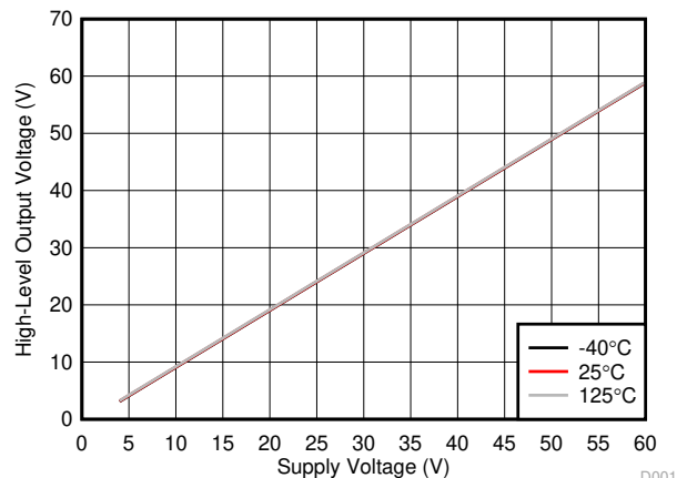
图 7-1. V_{OH} vs V_{SUP} and Temperature
