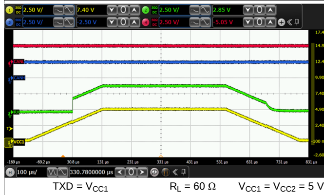
图 11. V_{OD(DOM)} Over V_{CC}
