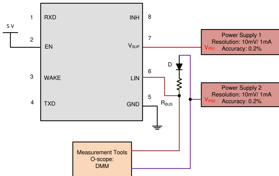
图 8-5. V SUP_NON_OP Param 11
