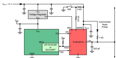
指挥官节点简化原理图 (1)
