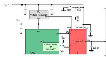
响应者节点简化原理图 (2)
