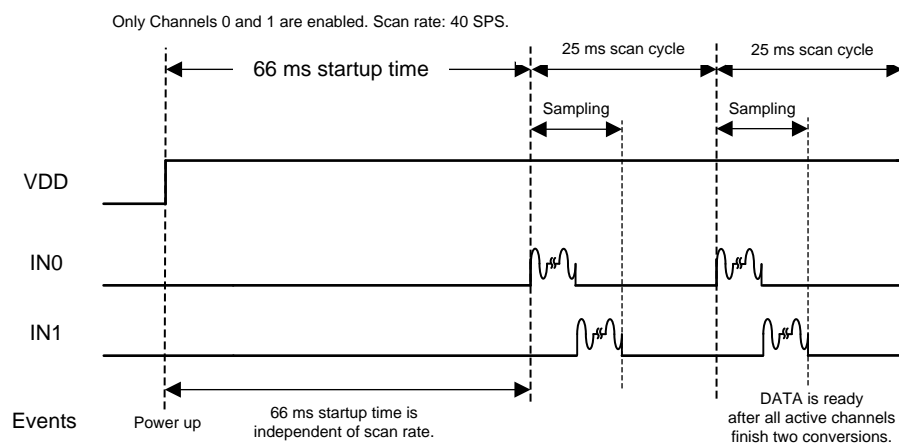
图 21. Power-On Timing
