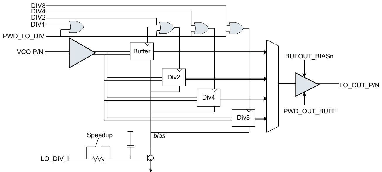
Figure 81. LO Divider
